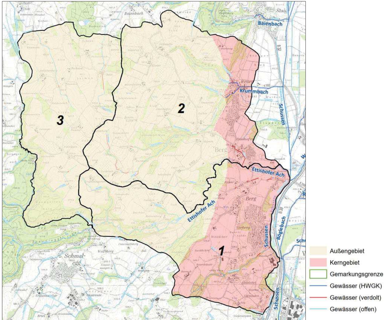
Abbildung 5.10 Außen- und Kerngebiet mit den Teileinzugsgebieten des Starkregenmodells für das Untersuchungsgebiet Berg
